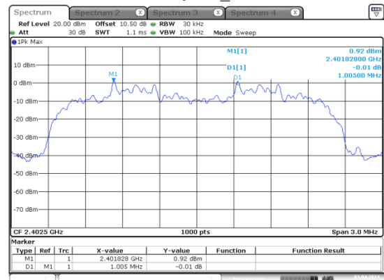
\pi/4 -DQPSK_Low
