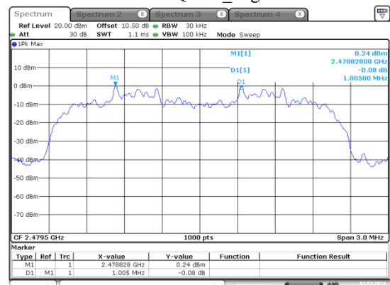
\pi/4 -DQPSK_High
