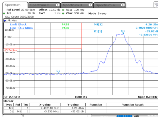
GFSK_Low_DH1
