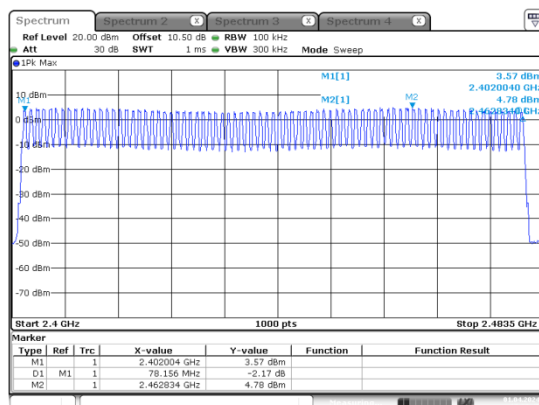
GFSK_Hopping_DH1
