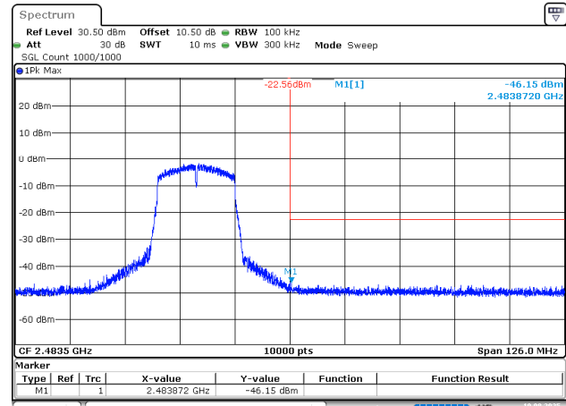
802.11n20_2462MHz
