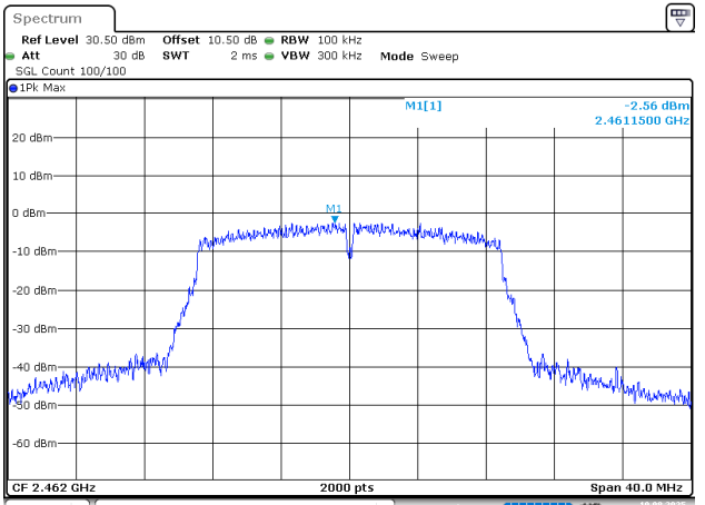
802.11n20_2462MHz
