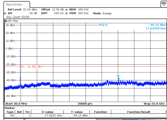
802.11n20_2437MHz
