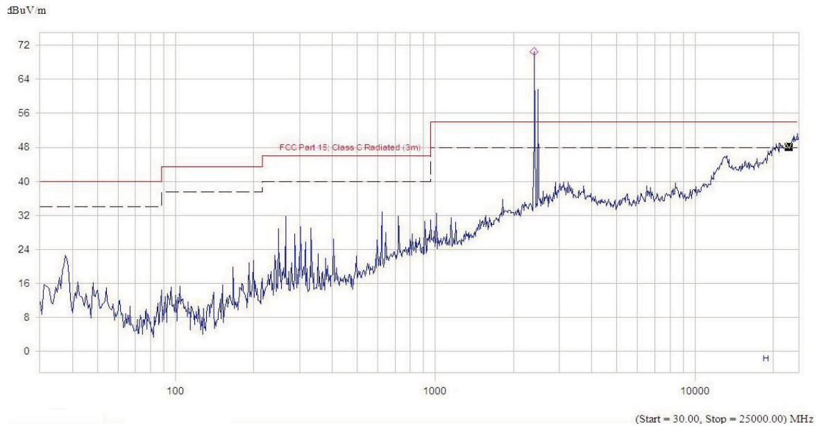
(Plot A.1: Antenna Horizontal)
