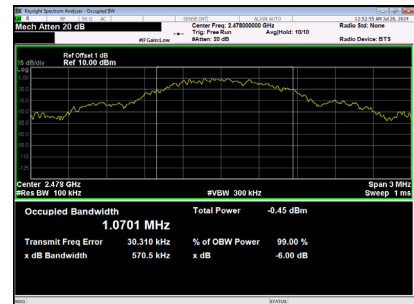
2478MHz
