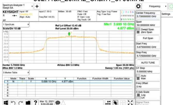
802.11ax_20MHz_Chain1_5700MHz_RU106_54
