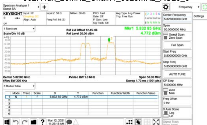
802.11ax_20MHz_Chain1_5825MHz_RU52_40
