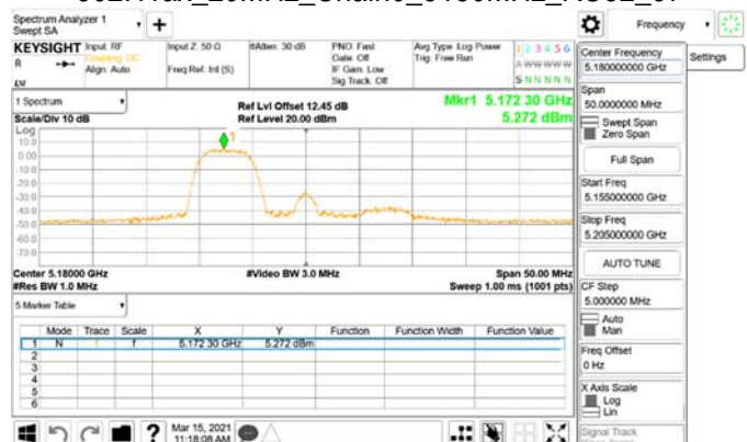
802.11ax_20MHz_Chain0_5180MHz_RU52_37
