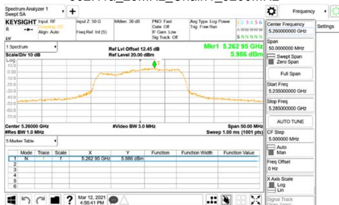
802.11a_20MHz_Chain1_5260MHz
