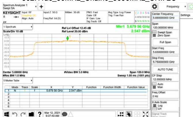
802.11ac_80MHz_Chain0_5690MHz_UNII 3
