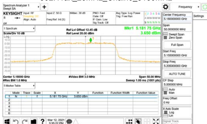
802.11ax_20MHz_Chain0_5180MHz
