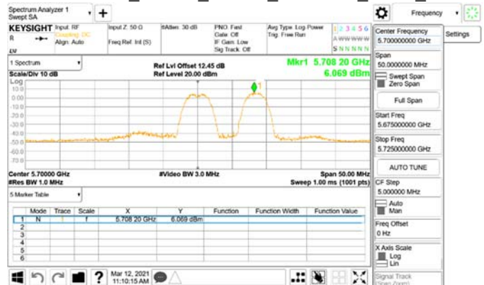
802.11ax_20MHz_Chain0_5700MHz_RU52_40
