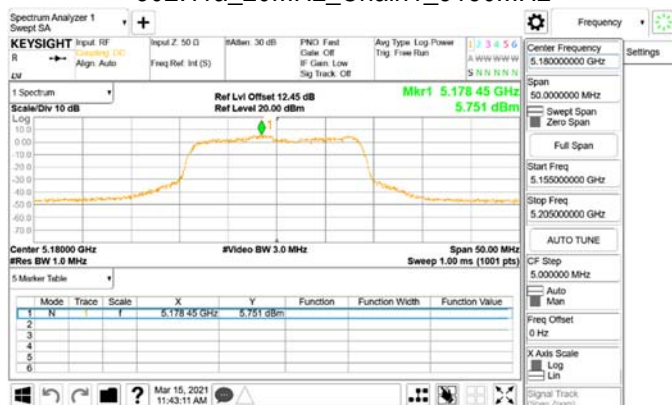
802.11a_20MHz_Chain1_5180MHz
