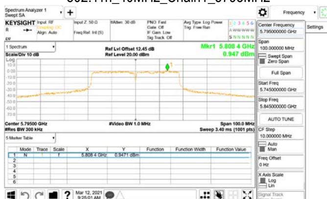
802.11n_40MHz_Chain1_5795MHz
