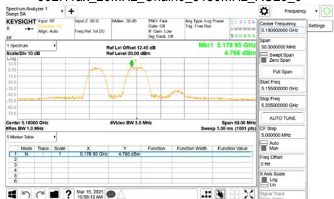
802.11ax_20MHz_Chain0_5180MHz_RU52_37
