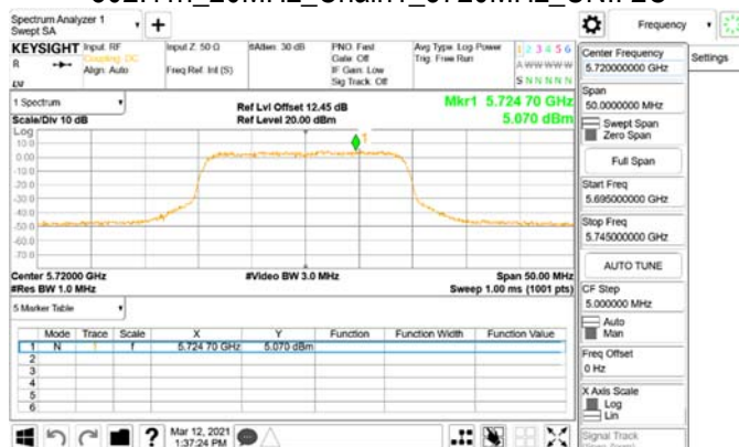
802.11n_20MHz_Chain1_5720MHz_UNII 3
