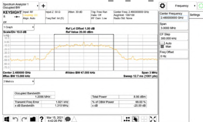
OBW 20dB \pi /4DQPSK_2M_DH5_2480MHz
