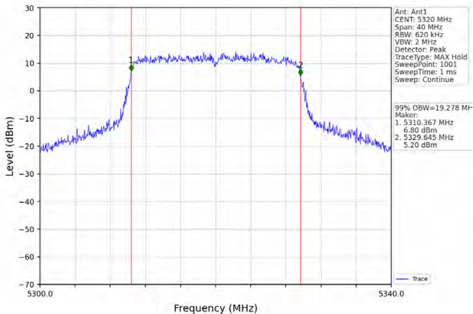
802.11ax(HEW20)_HCH_5320MHz_RU242_Left_Ant1_NTNV
