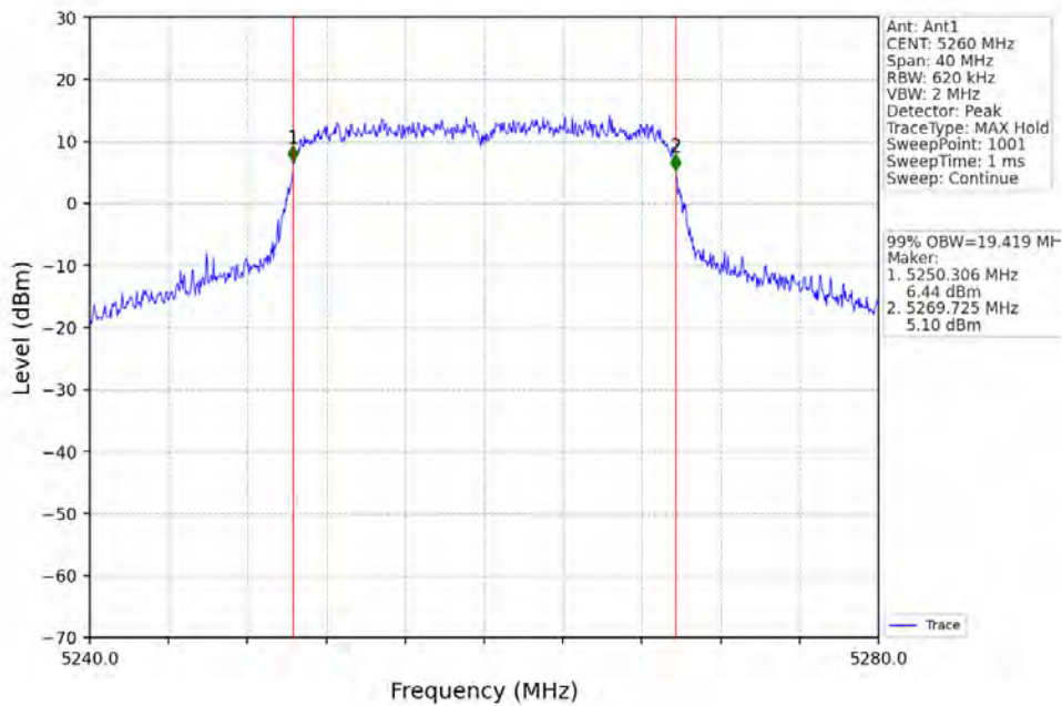
802.11ax(HEW20)_LCH_5260MHz_RU242_Left_Ant1_NTNV
