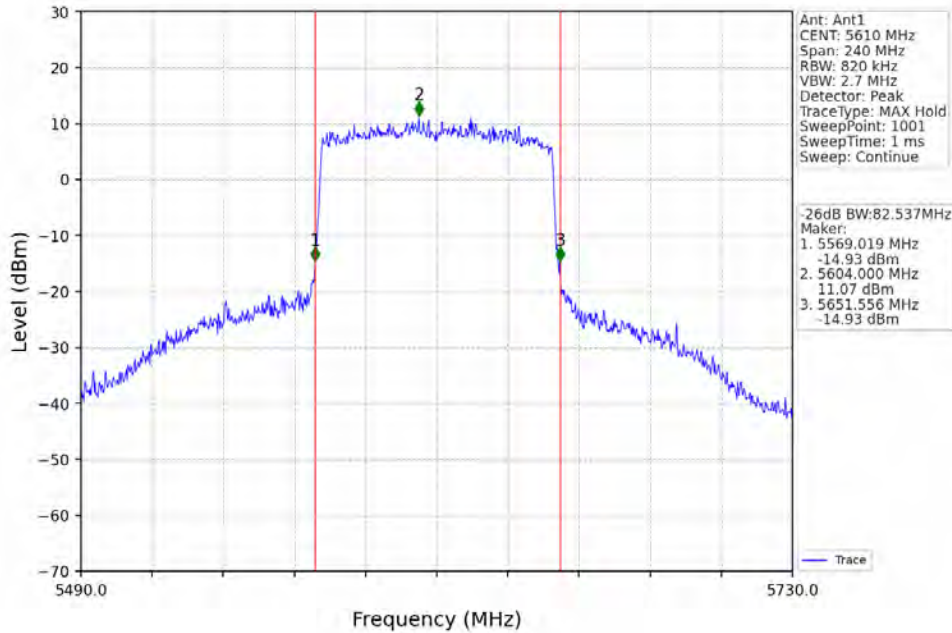
802.11ax(HEW160)_MCH_5570MHz_2xRU996_Left_Ant1_NTNV
