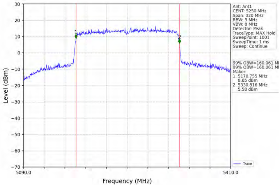
802.11ax(HEW160)_MCH_5250MHz_2xRU996_Left_Ant1_NTNV
