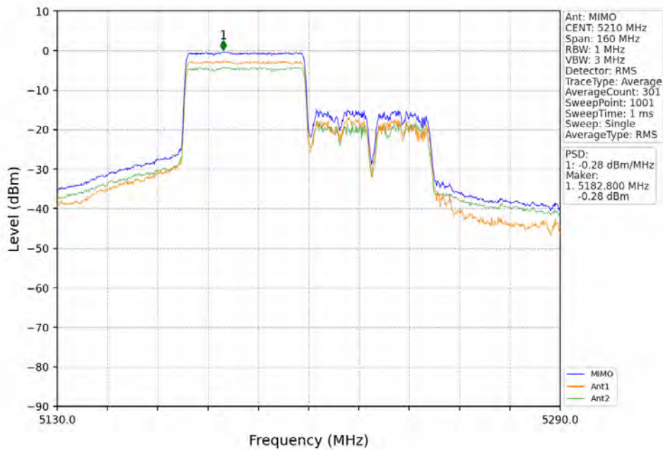
802.11ax(HEW80)_MCH_5210MHz_RU484_Left_MIMO_NTNV
