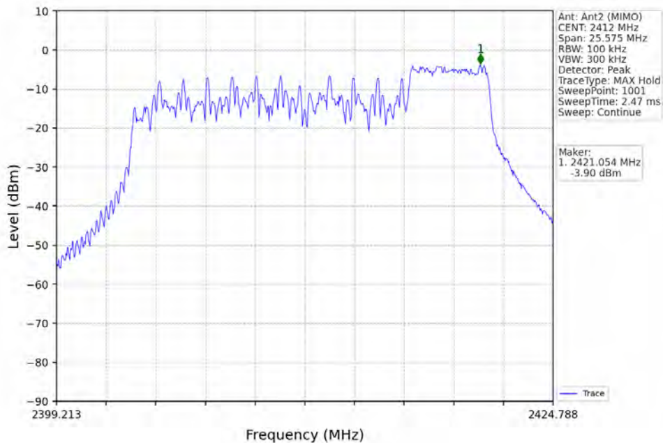
802.11ax(HEW20)_LCH_2412MHz_RU52_Right_Ant2 (MIMO)_NTNV
