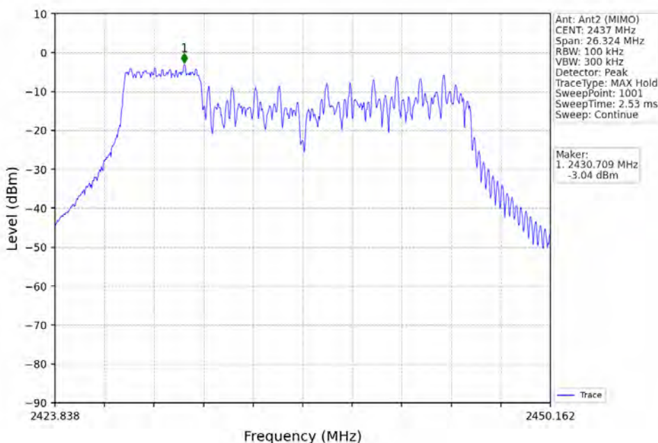
802.11ax(HEW20)_MCH_2437MHz_RU52_Left_Ant2 (MIMO)_NTNV
