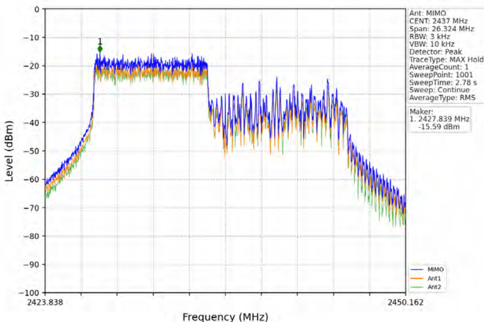
802.11ax(HEW20)_MCH_2437MHz_RU106_Left_MIMO_NTNV
