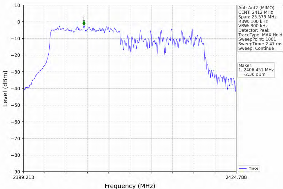
802.11ax(HEW20)_LCH_2412MHz_RU106_Left_Ant2 (MIMO)_NTNV
