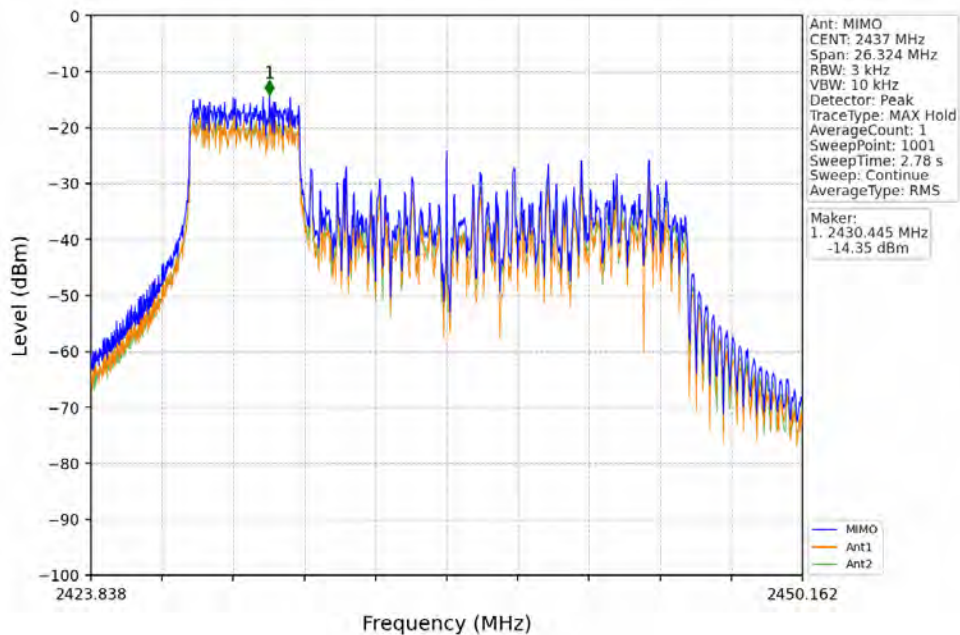
802.11ax(HEW20)_MCH_2437MHz_RU52_Left_MIMO_NTNV
