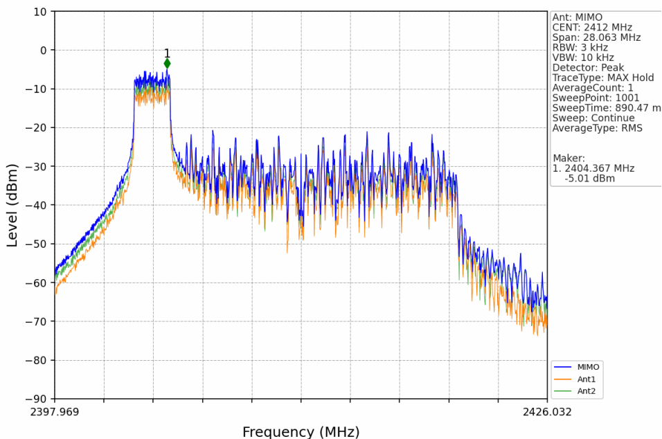
802.11ax(HEW20)_LCH_2412MHz_RU52_Left_Ant1 (MIMO)_NTNV
