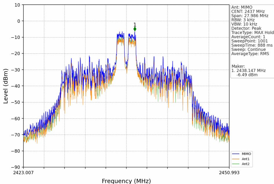
802.11ax(HEW20)_MCH_2437MHz_RU52_Mid_Ant1 (MIMO)_NTNV
