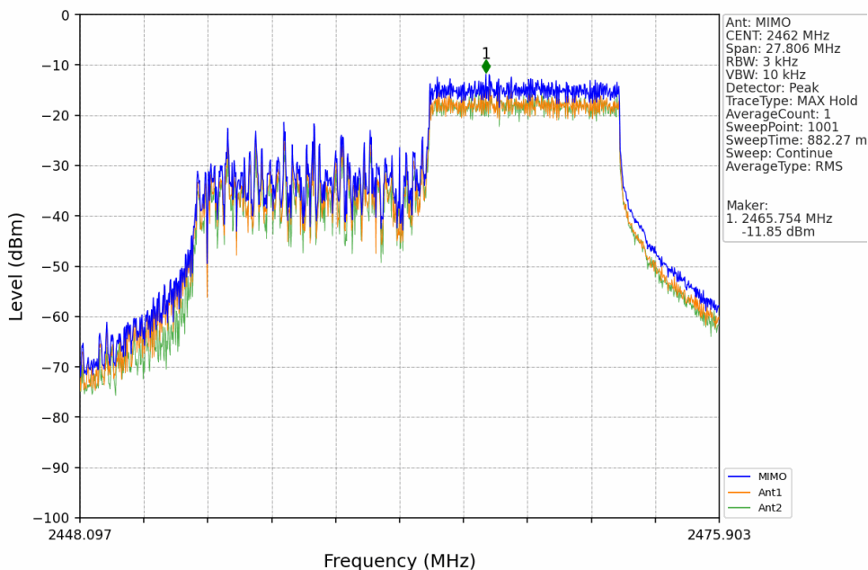
802.11ax(HEW20)_HCH_2462MHz_RU242_Left_Ant1 (MIMO)_NTNV
