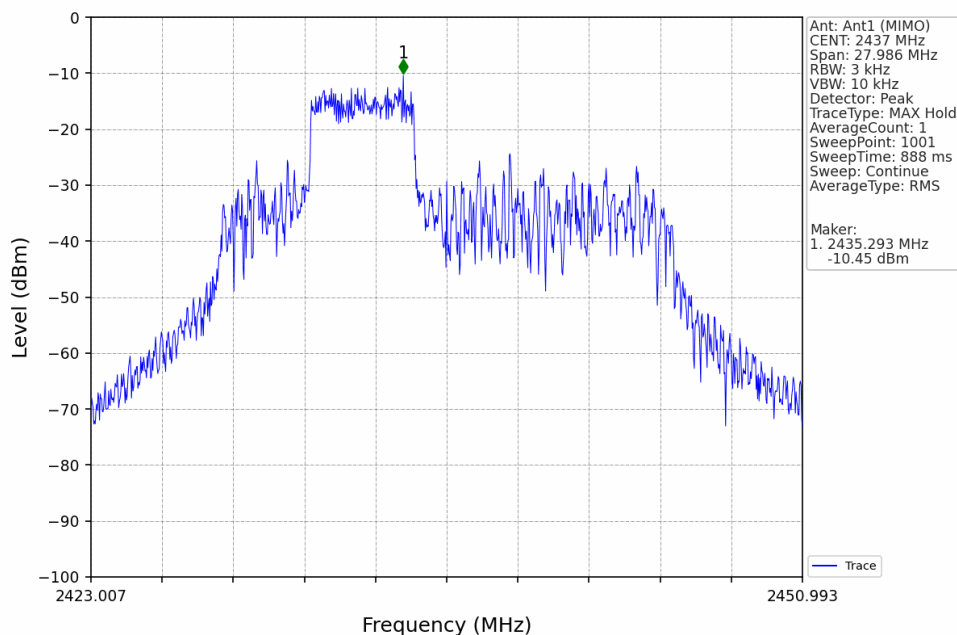
802.11ax(HEW20)_MCH_2437MHz_RU52_Mid_Ant1 (MIMO)_NTNV
