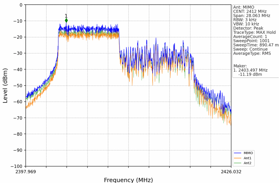
802.11ax(HEW20)_LCH_2412MHz_RU242_Left_Ant1 (MIMO)_NTNV
