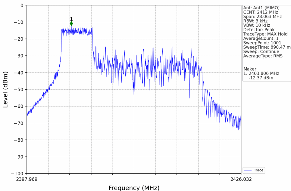
802.11ax(HEW20)_LCH_2412MHz_RU52_Left_Ant1 (MIMO)_NTNV
