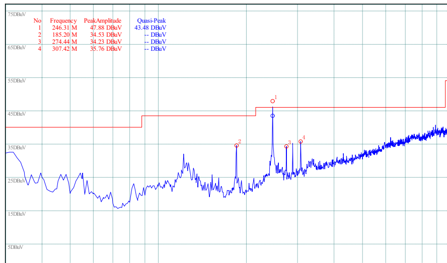
(Plot A: Test Antenna Vertical)
