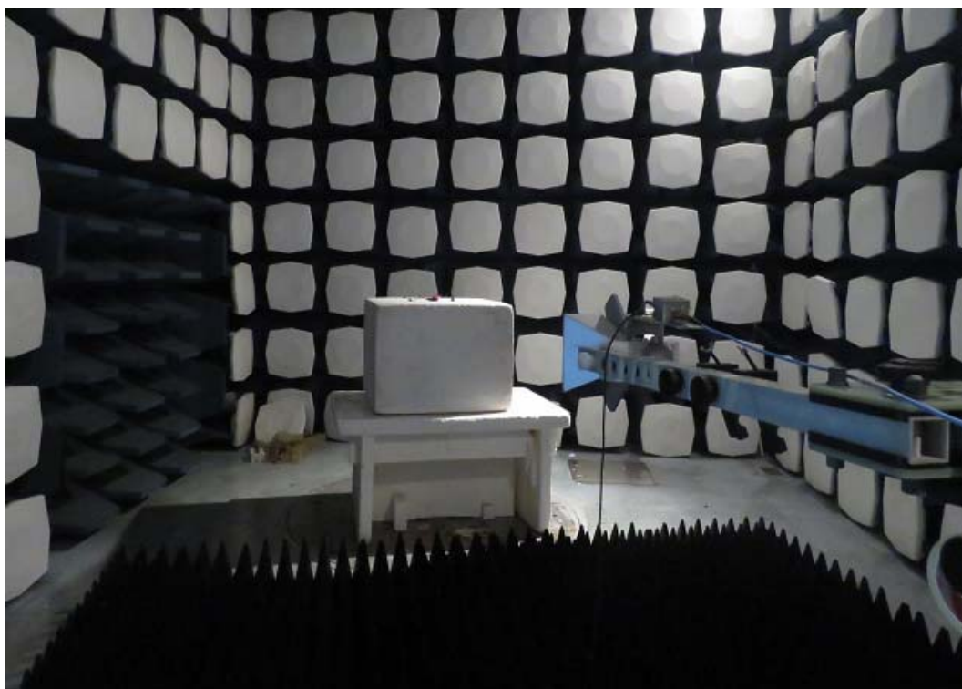
1GHz-18GHz
