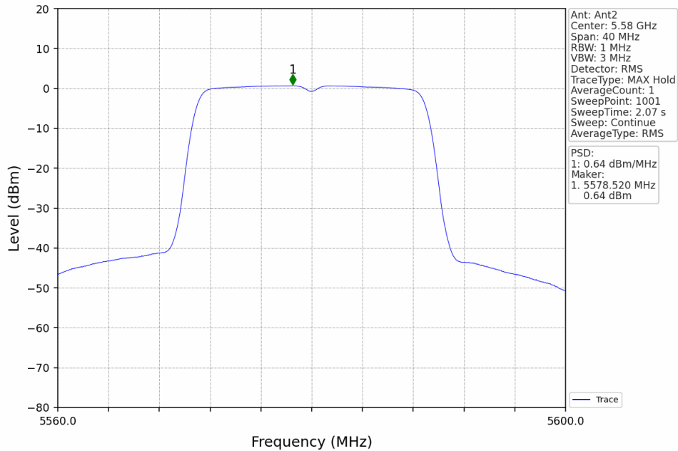
802.11n(HT20)_MCH_5580MHz_MIMO_NTNV
