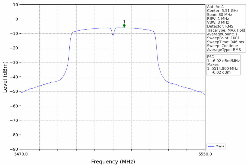
802.11n(HT40)_LCH_5510MHz_Ant1_NTNV
