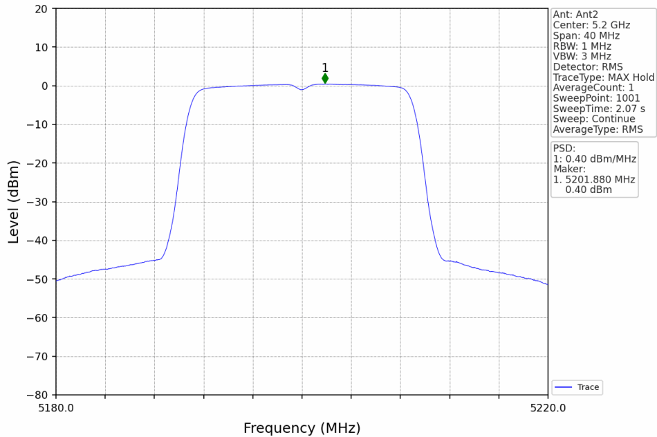
802.11n(HT20)_MCH_5200MHz_MIMO_NTNV
