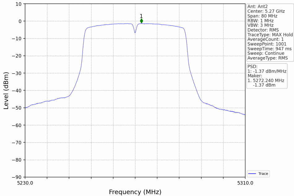
802.11n(HT40)_LCH_5270MHz_MIMO_NTNV
