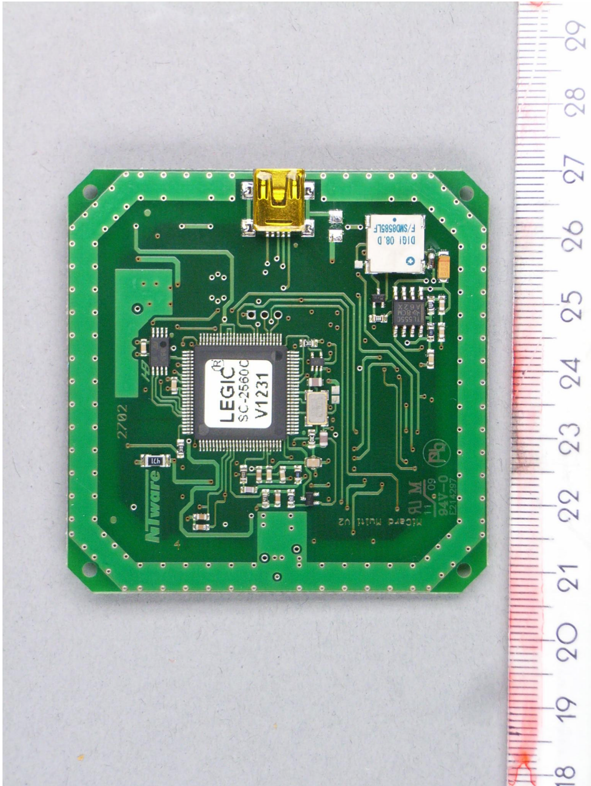
91053eut2.jpg MiCard V2 Multi, PCB rear view
