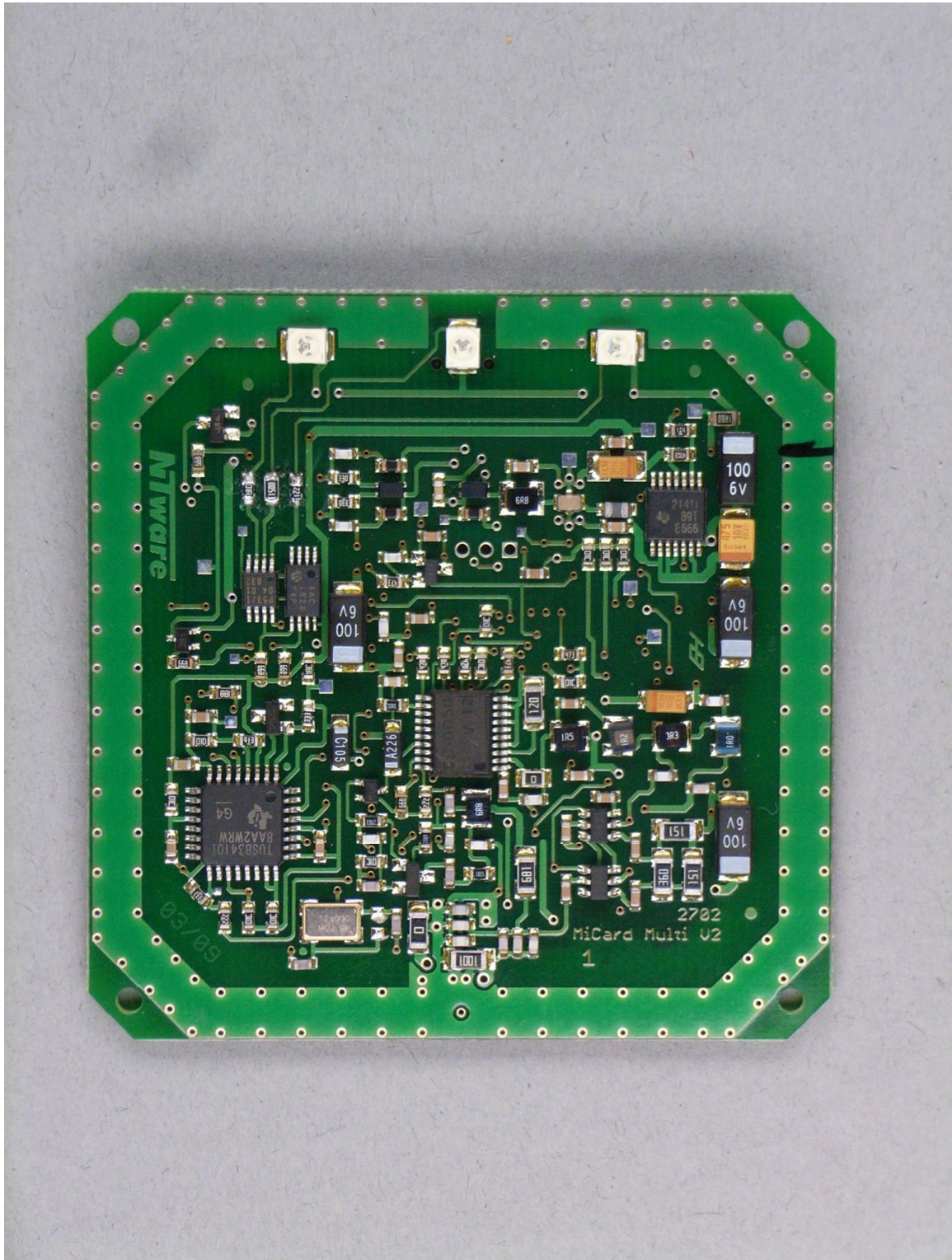
91053eut1.jpg MiCard V2 Multi, PCB top view
