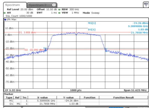
n20_5320MHz_Chain 0
