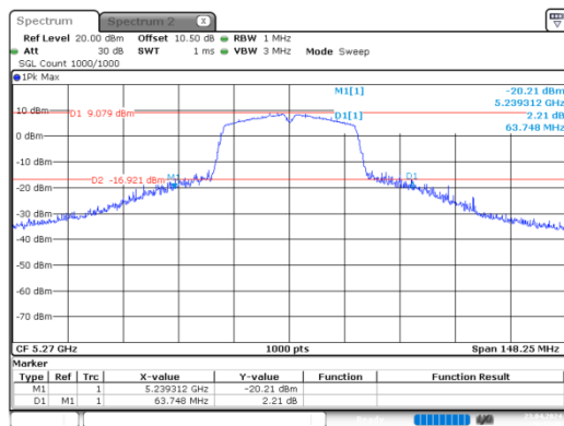
n40_5270MHz_Chain 0
