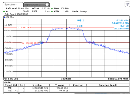
a_5280MHz_Chain 0
