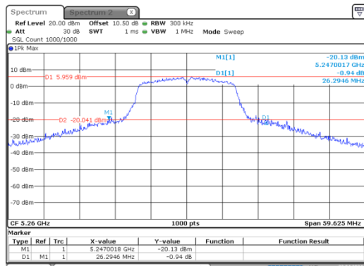
a_5260MHz_Chain 0
