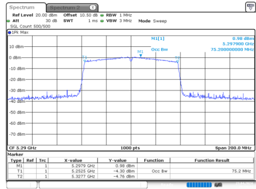
ac80_5290MHz_Chain 0
