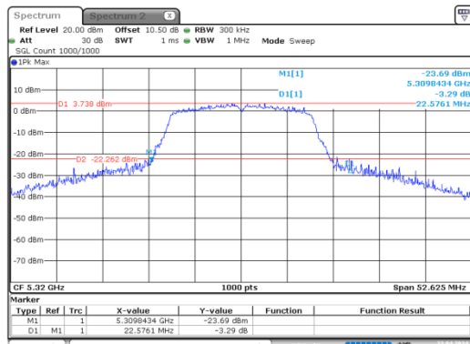
a_5320MHz_Chain 0
