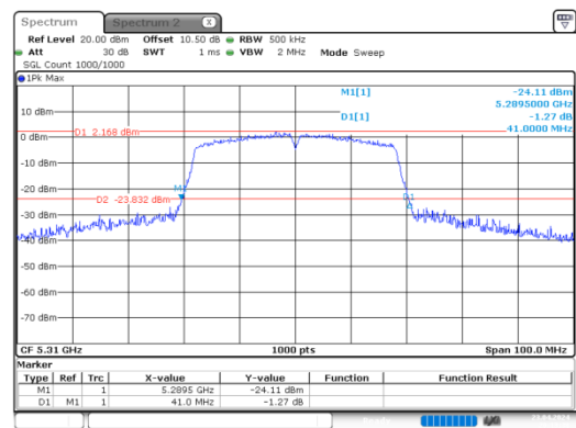
n40_5310MHz_Chain 0
