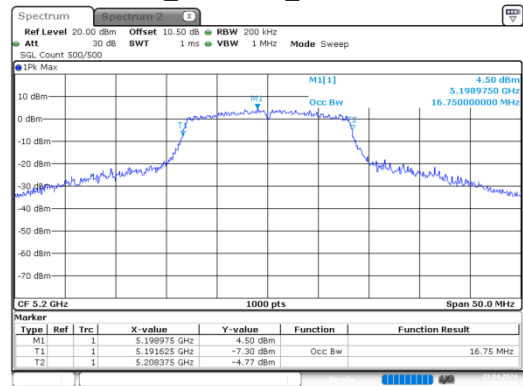
a_5200MHz_Chain 0
