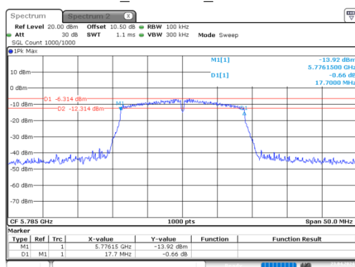
n20_ 5785MHz_Chain 0
