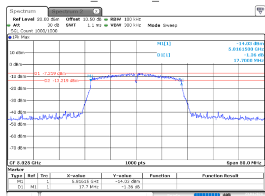
n20_ 5825MHz_Chain 0
