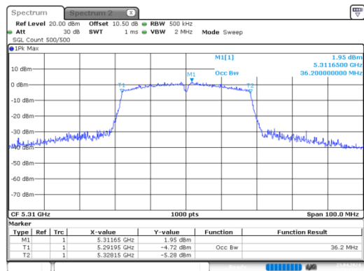
n40_5310MHz_Chain 0
