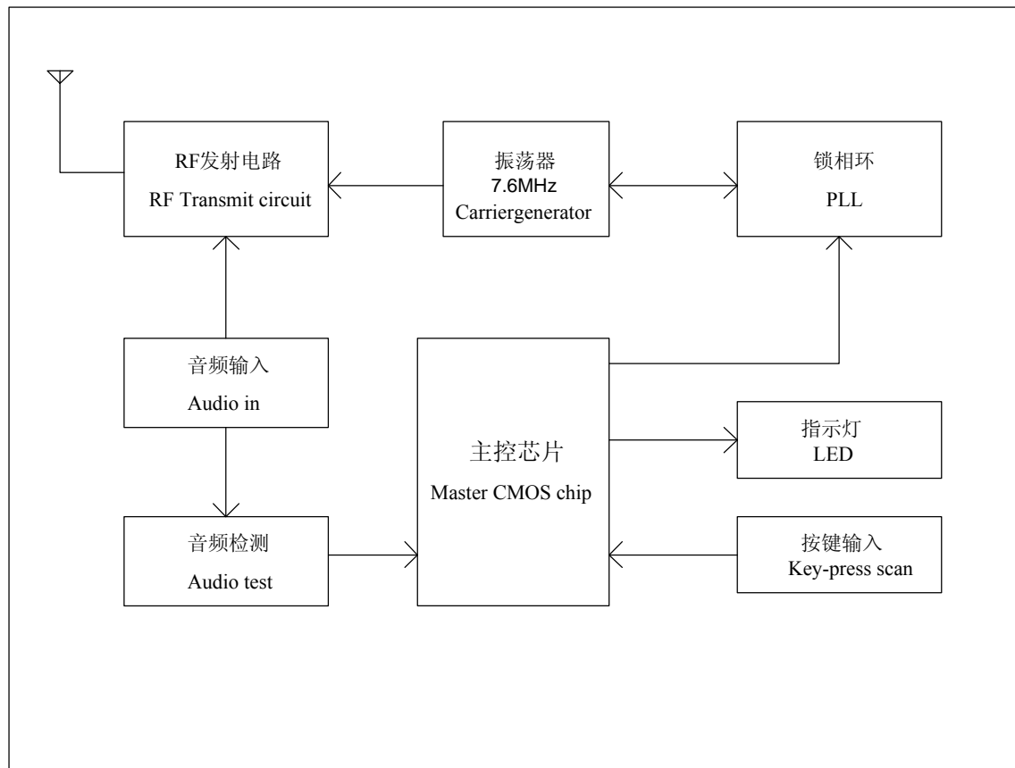
电路方框图 Circuit diagram
