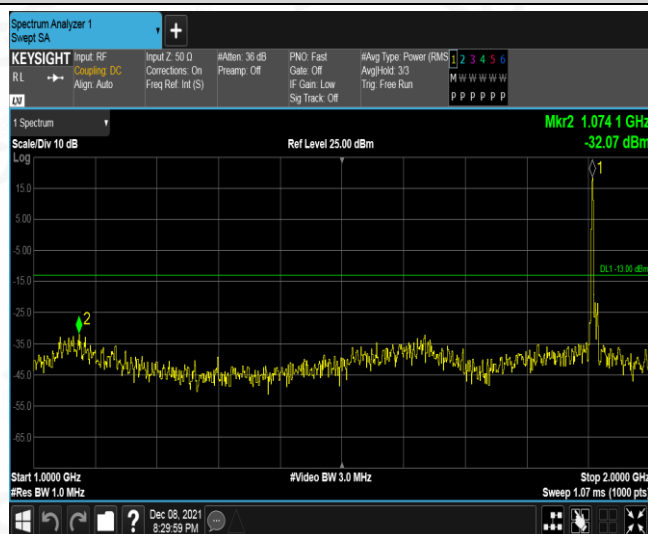
Band2-5MHz-16QAM-19175-1RB#0-Range2:1000~2000MHz
