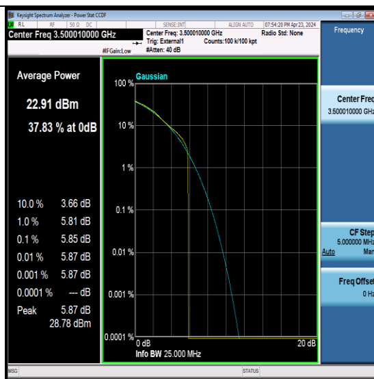
NTNV- N78-3450-3550-PC2-30-20-M-CP-QPSK-Edge_1RB_Left-PASS
