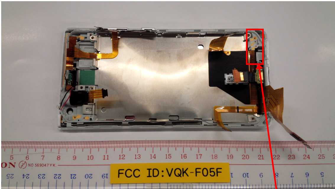
WWAN ANTENNA
