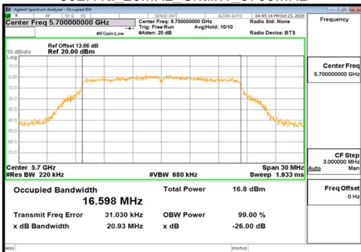
802.11a 20MHz_Chain1_5700MHz
