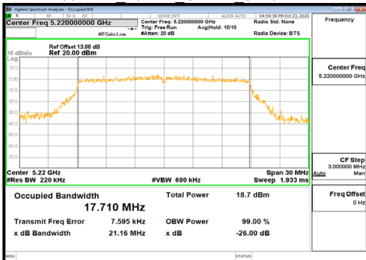
802.11n 20MHz Chain1 5220MHz
