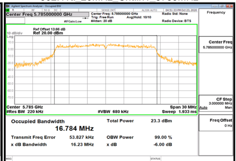
802.11a 20MHz_Chain1_5785MHz
