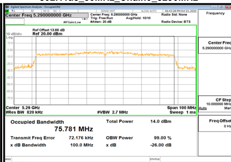
802.11ac_80MHz_Chain0_5290MHz
