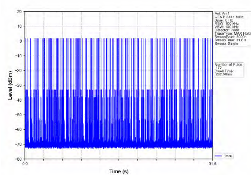
8DPSK_3DH3_HOPP_Ant1_NTNV
