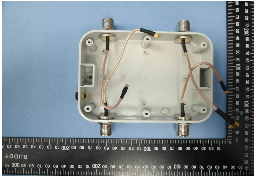
EUT Photo (19)
