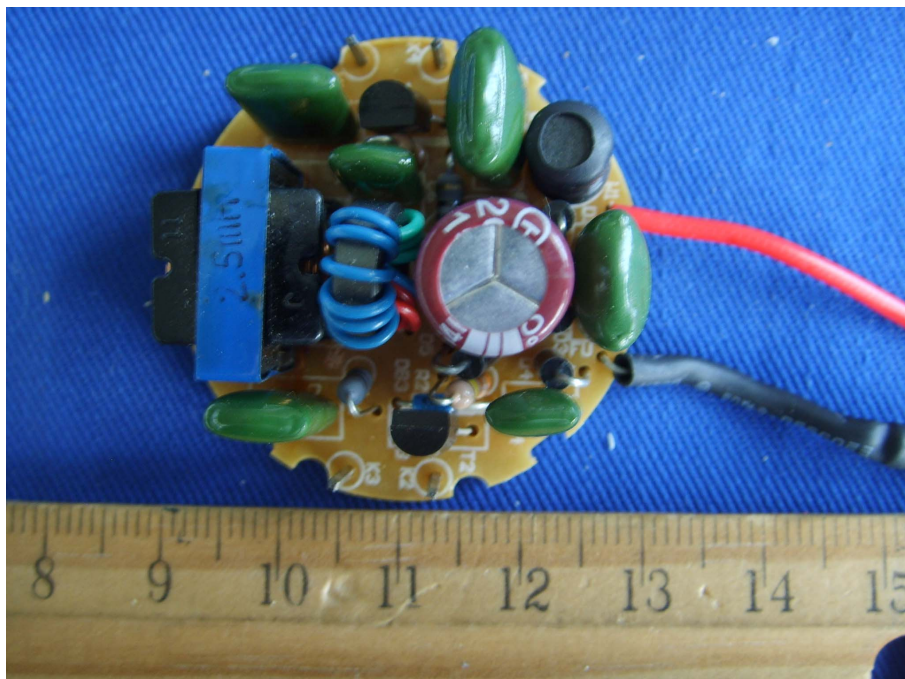
EUT –Components View (MSG13W)
