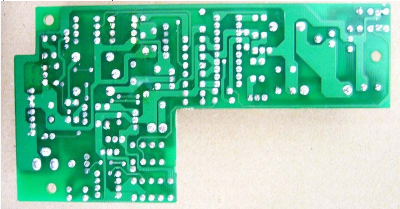
(SCS36-12BAT BOTTOM)
