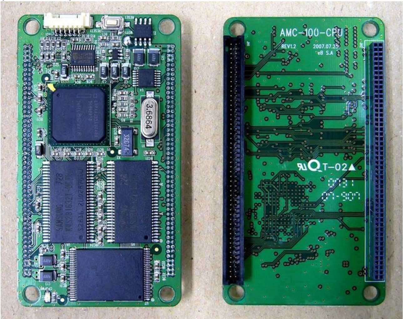
(AMC-100 CPU)
