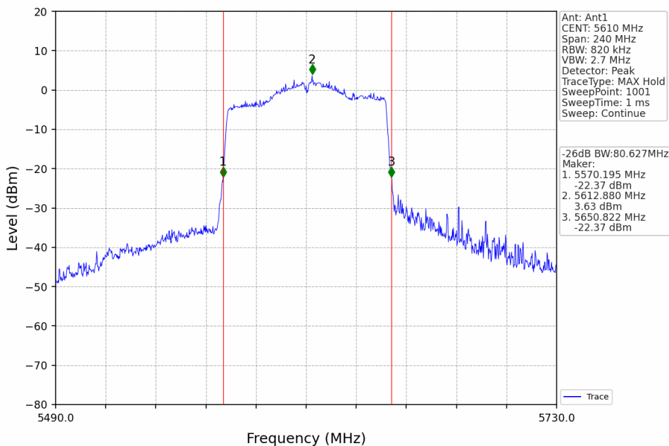
802.11ac(VHT80)_HCH_5610MHz_Ant1_NTNV
