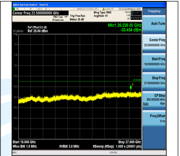
Band7_20MHz_16QAM_20850_100RB#0_18000~27000_18000~27000
