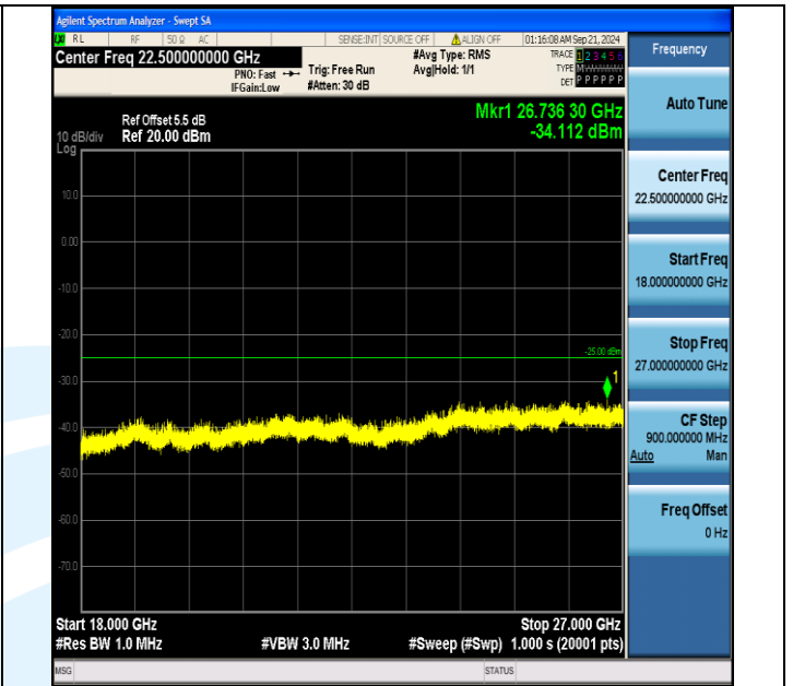
Band7_20MHz_QPSK_21350_1RB#0_18000~27000_18000~27000
