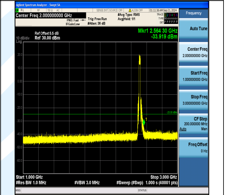
Band7_20MHz_QPSK_20850_100RB#0_1000~3000_1000~3000
