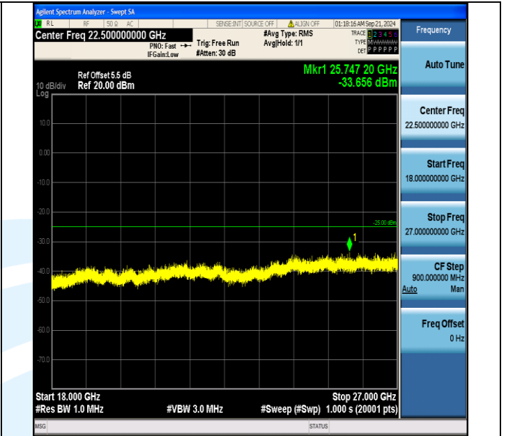
Band7_20MHz_QPSK_21350_100RB#0_18000~27000_18000~27000
