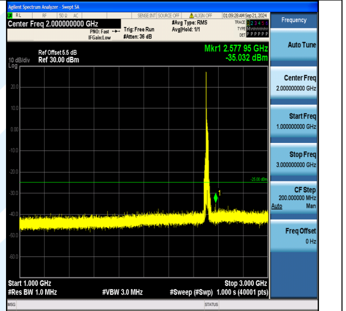
Band7_20MHz_QPSK_20850_1RB#0_1000~3000_1000~3000
