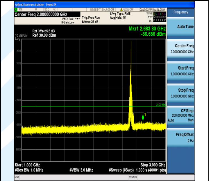
Band7_20MHz_QPSK_20850_1RB#99_1000~3000_1000~3000
