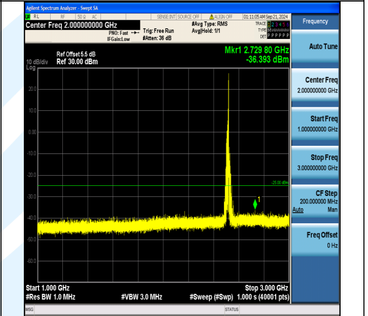
Band7_20MHz_16QAM_20850_1RB#99_1000~3000_1000~3000
