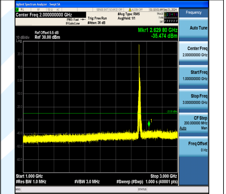
Band7_20MHz_16QAM_20850_1RB#0_1000~3000_1000~3000
