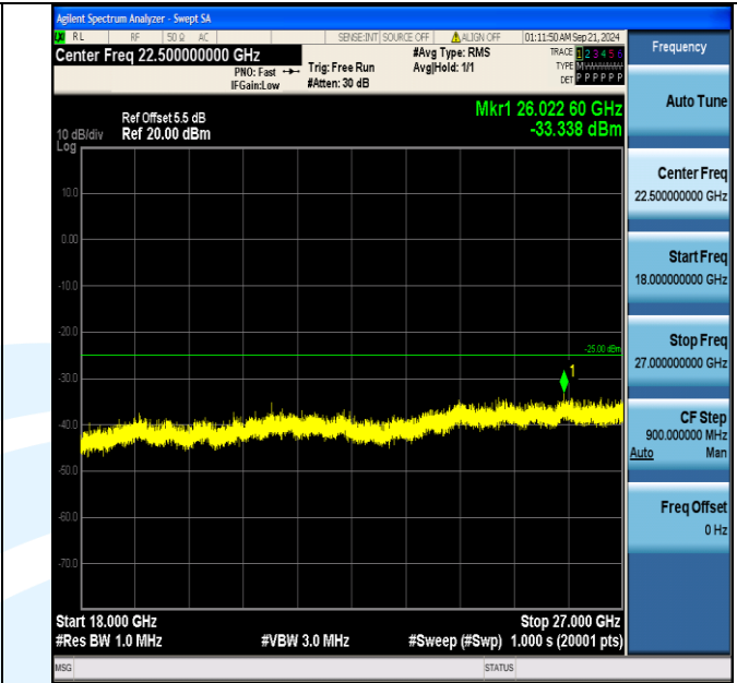
Band7_20MHz_QPSK_20850_100RB#0_18000~27000_18000~27000
