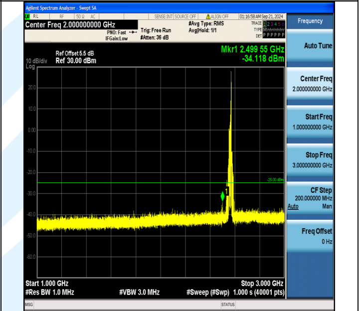
Band7_20MHz_QPSK_21350_1RB#99_1000~3000_1000~3000
