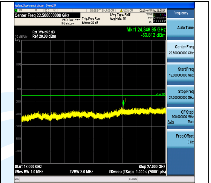
Band7_20MHz_QPSK_20850_1RB#99_18000~27000_18000~27000
