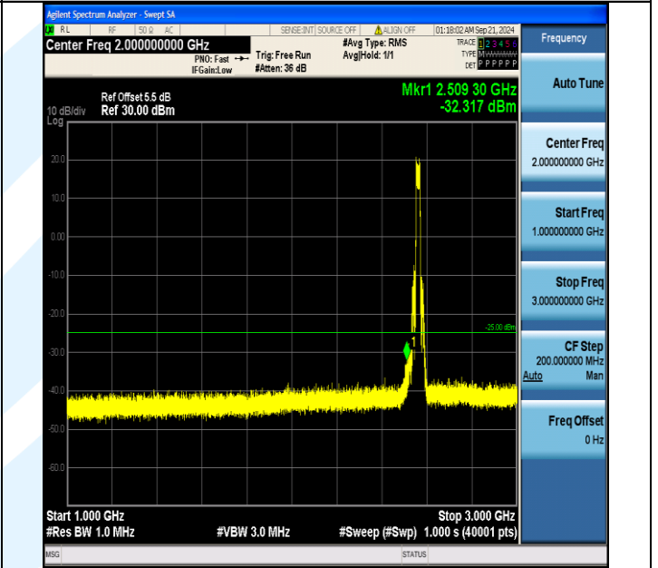
Band7_20MHz_QPSK_21350_100RB#0_1000~3000_1000~3000
