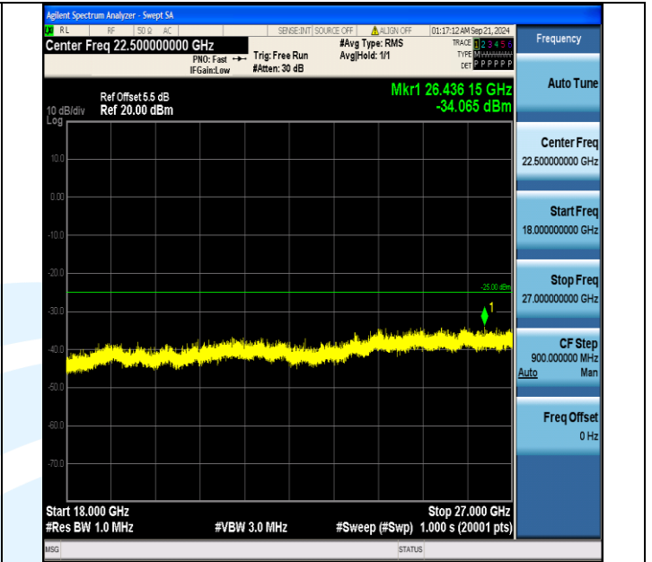
Band7_20MHz_QPSK_21350_1RB#99_18000~27000_18000~27000
