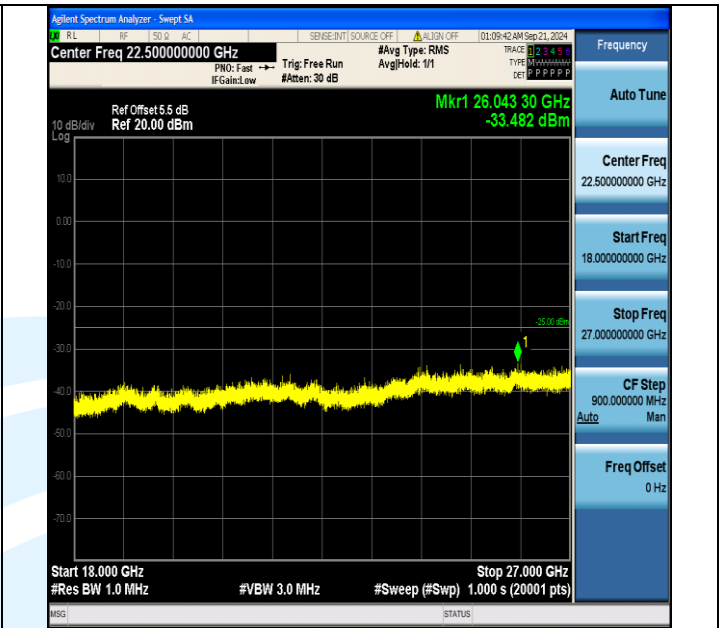
Band7_20MHz_QPSK_20850_1RB#0_18000~27000_18000~27000
