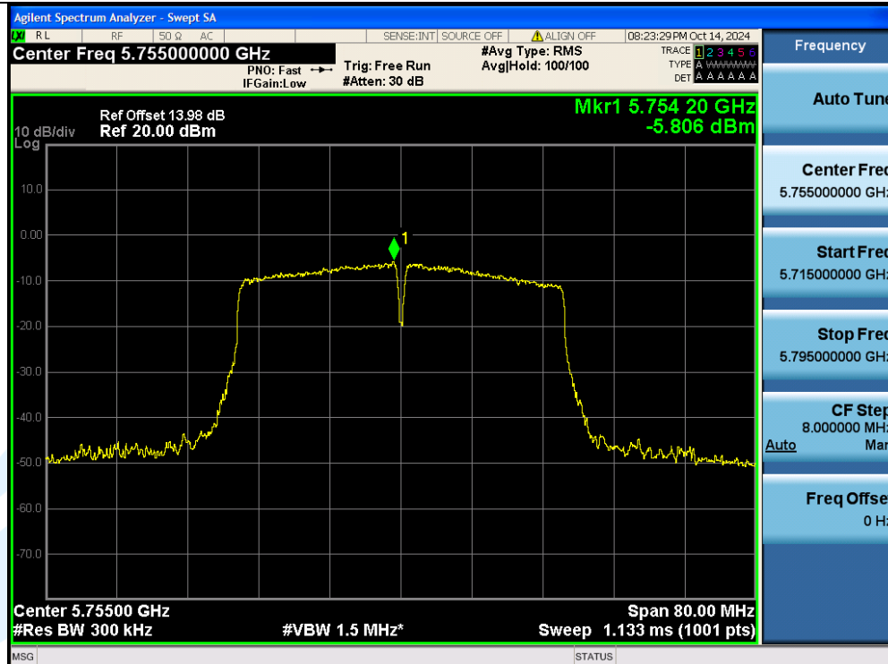
11N40SISO-Ant1-5755-PASS
