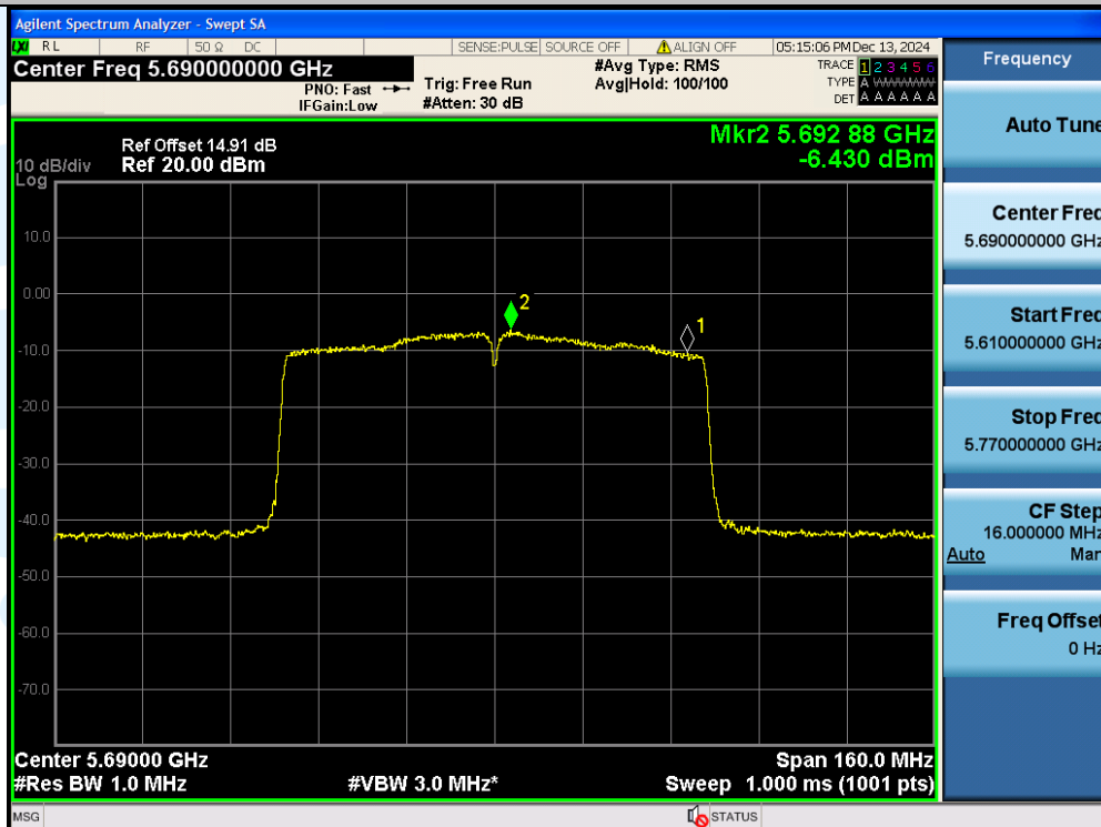
11AC80SISO-Ant1-5690_UNII-2C-PASS
