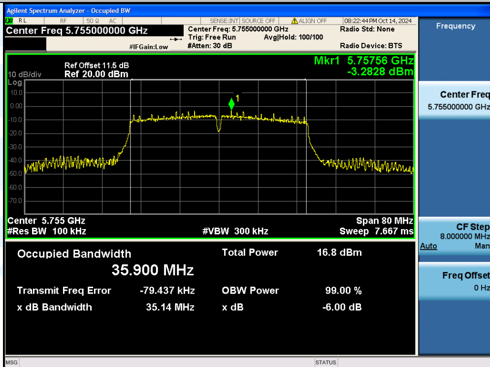
11N40SISO-Ant1-5755-PASS
