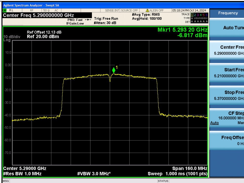
11AC80SISO-Ant1-5290-PASS
