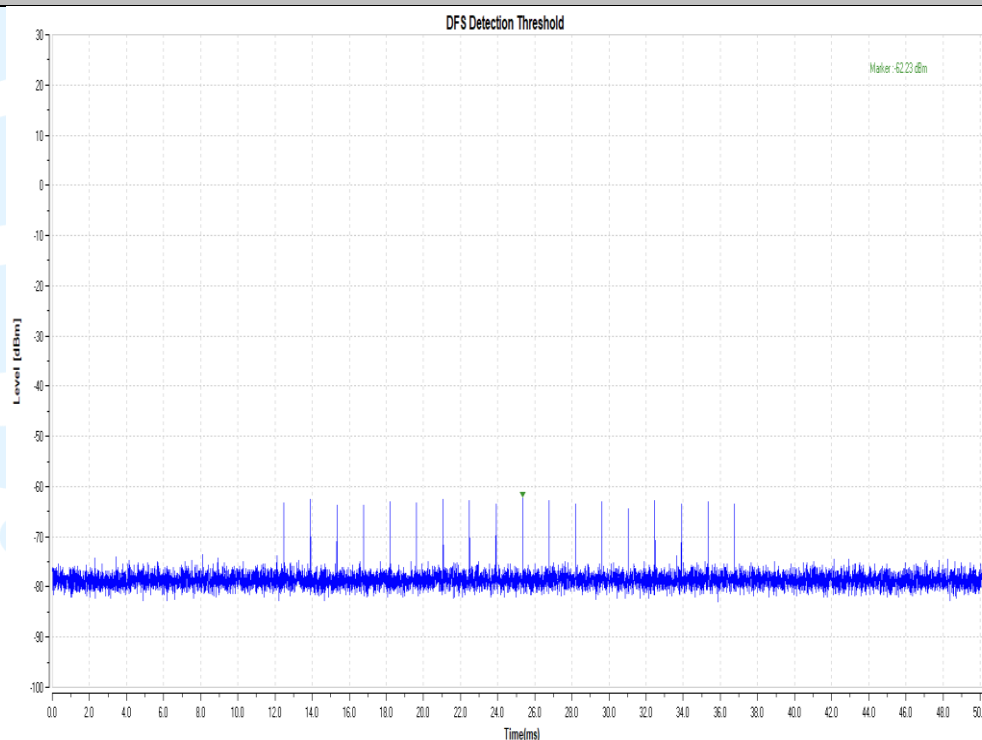
11AC80SISO-5530-Type0-PASS
