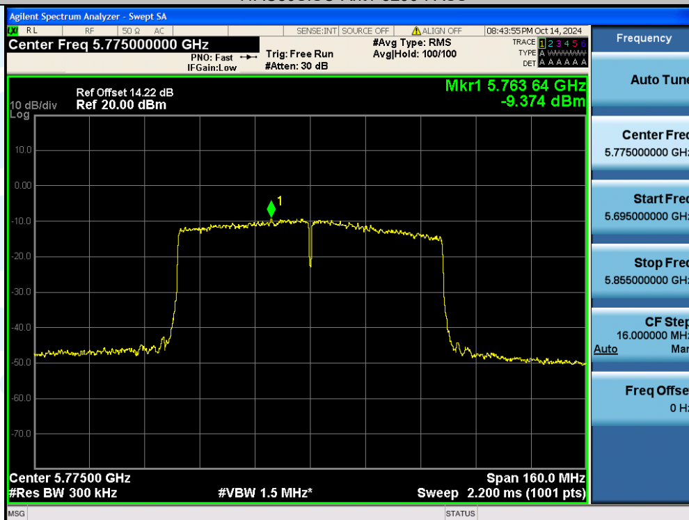
11AC80SISO-Ant1-5775-PASS
