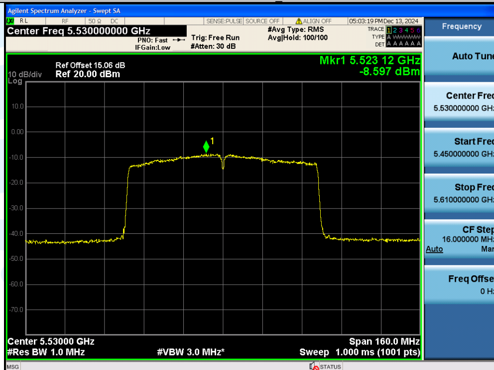
11AC80SISO-Ant1-5530-PASS
