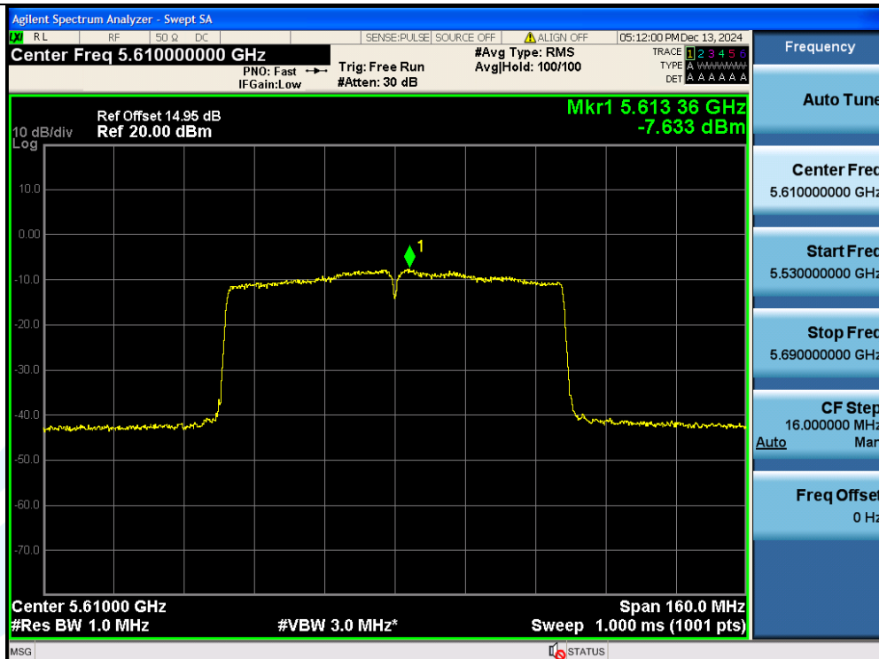
11AC80SISO-Ant1-5610-PASS
