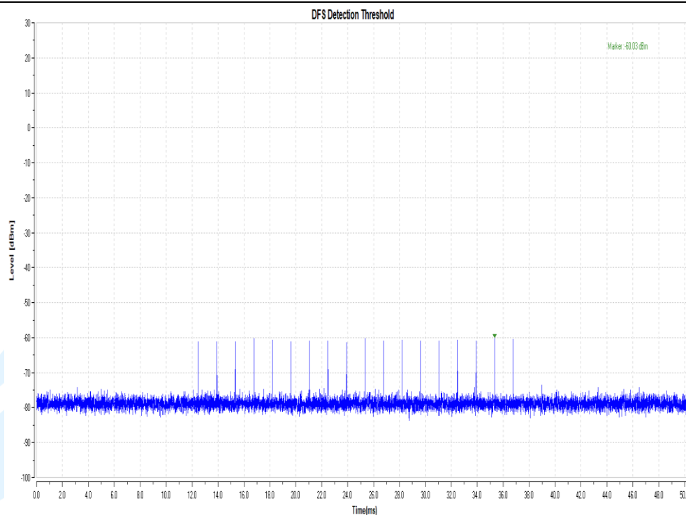
11AC80SISO-5290-Type0-PASS
