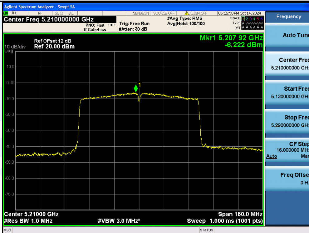
11AC80SISO-Ant1-5210-PASS
