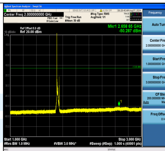
Band4 20MHz QPSK 20050 1RB#0 1000~3000 1000~3000
