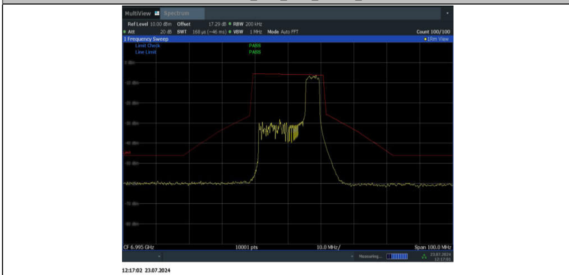
11AX20SISO_Ant2_6995_52Tone_RU40
