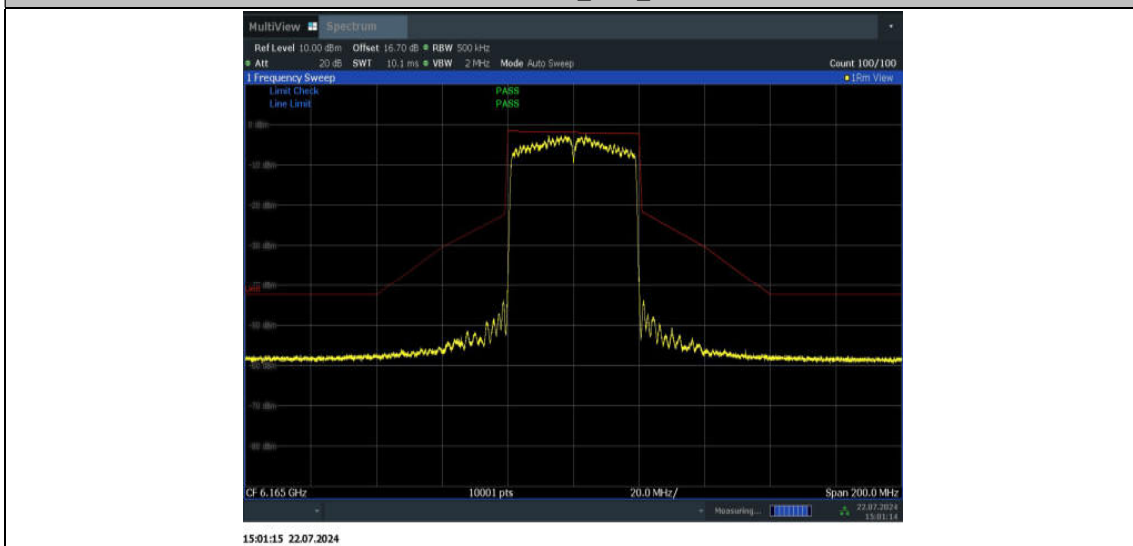
11AX40SISO_Ant2_6165
