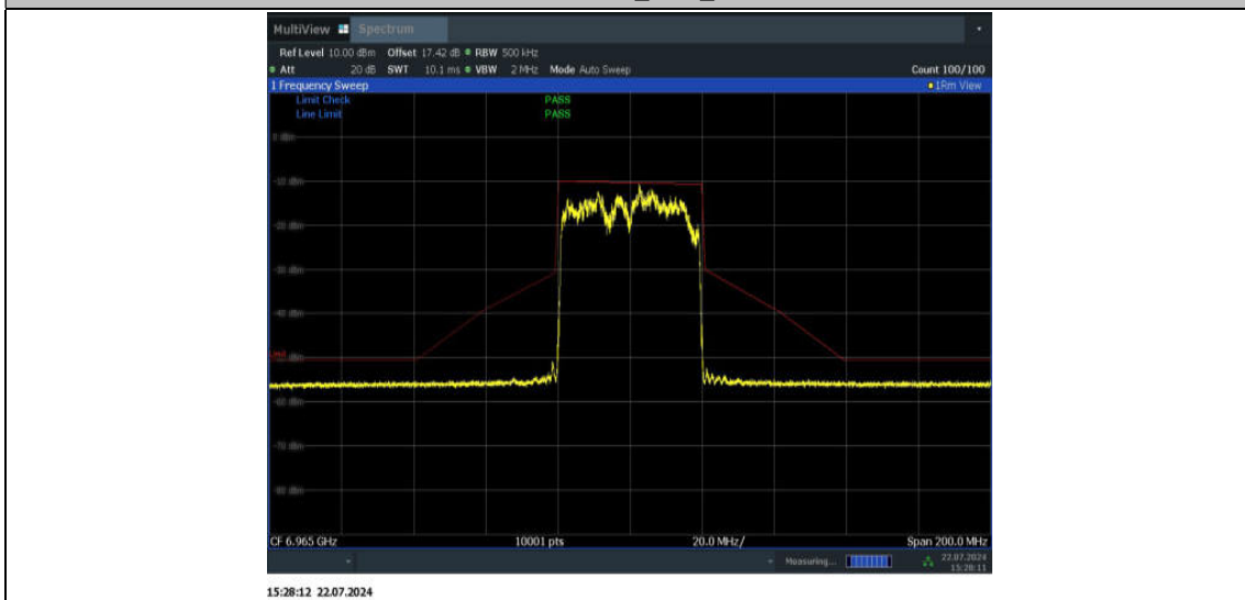
11AX40SISO_Ant2_6965
