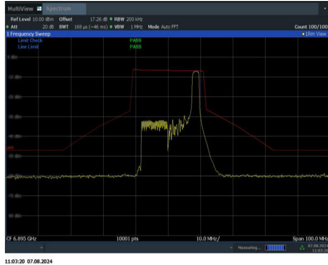
11AX20SISO_Ant2_6895_52Tone_RU40
