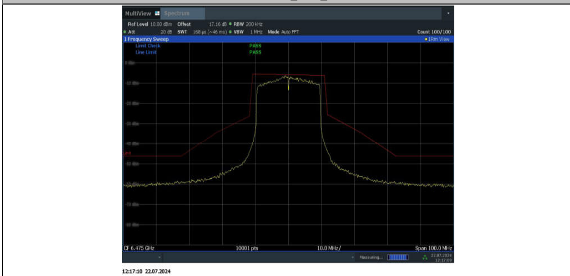
11AX20SISO_Ant2_6475
