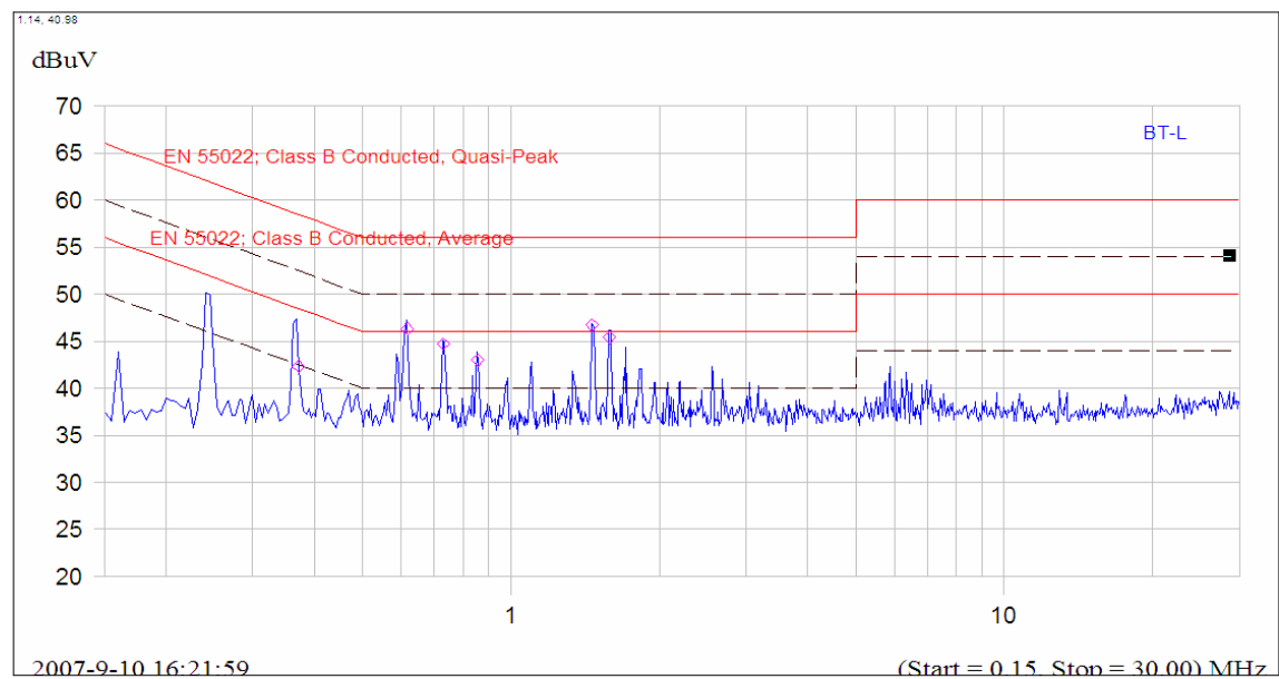
(Plot B: L Phase)
