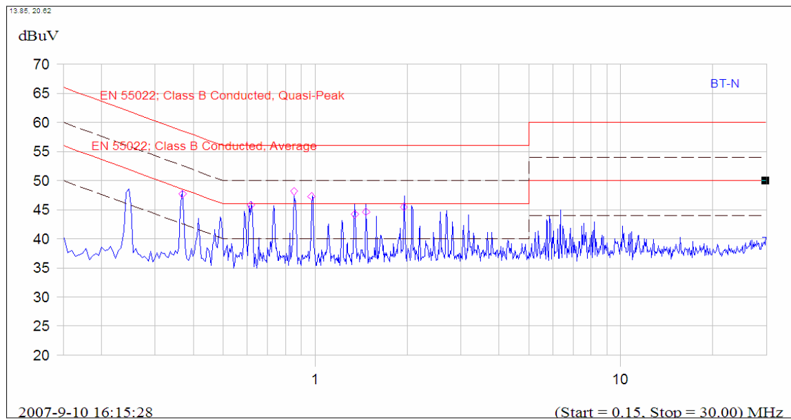
(Plot A: N Phase)
