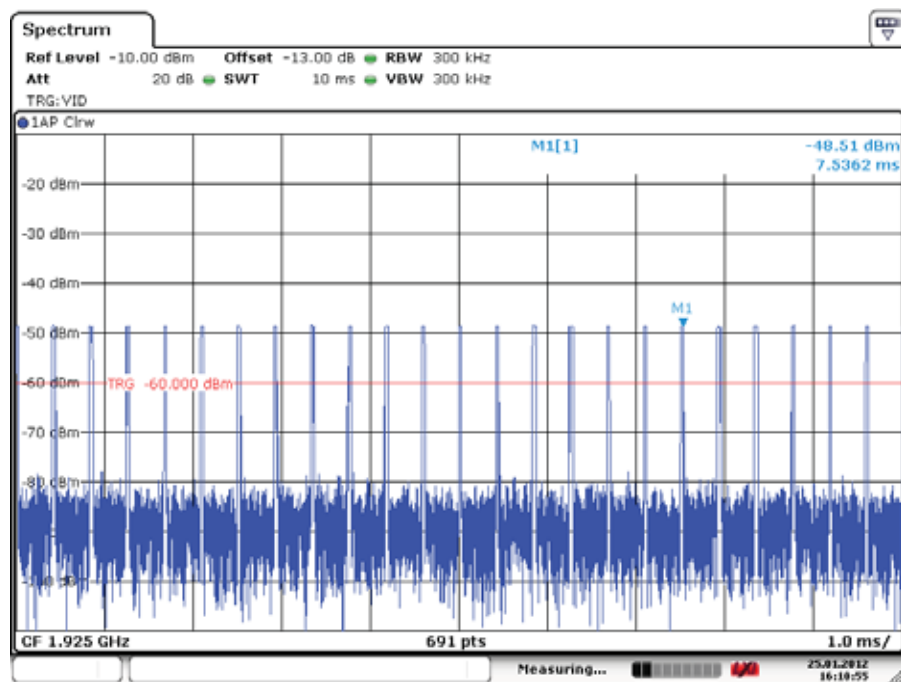
35 µs Pulses
