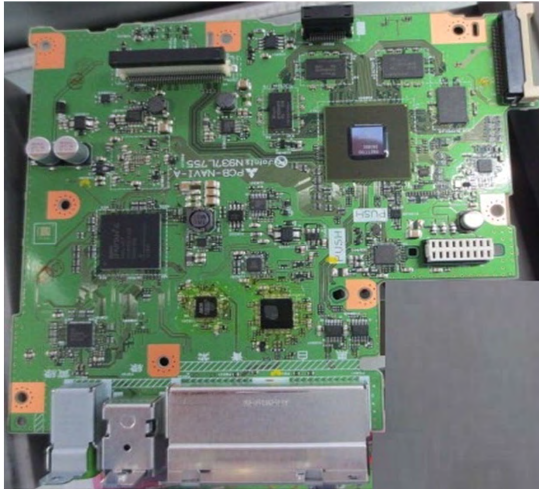
1. PCB-NAVI (PCB-NAVI-A) C-side
