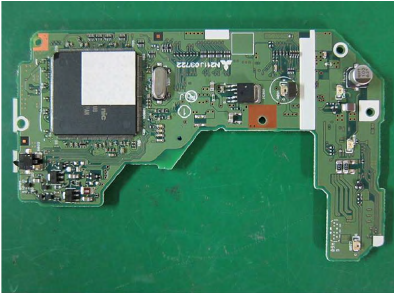
20. PCB SingleDeck S-side
