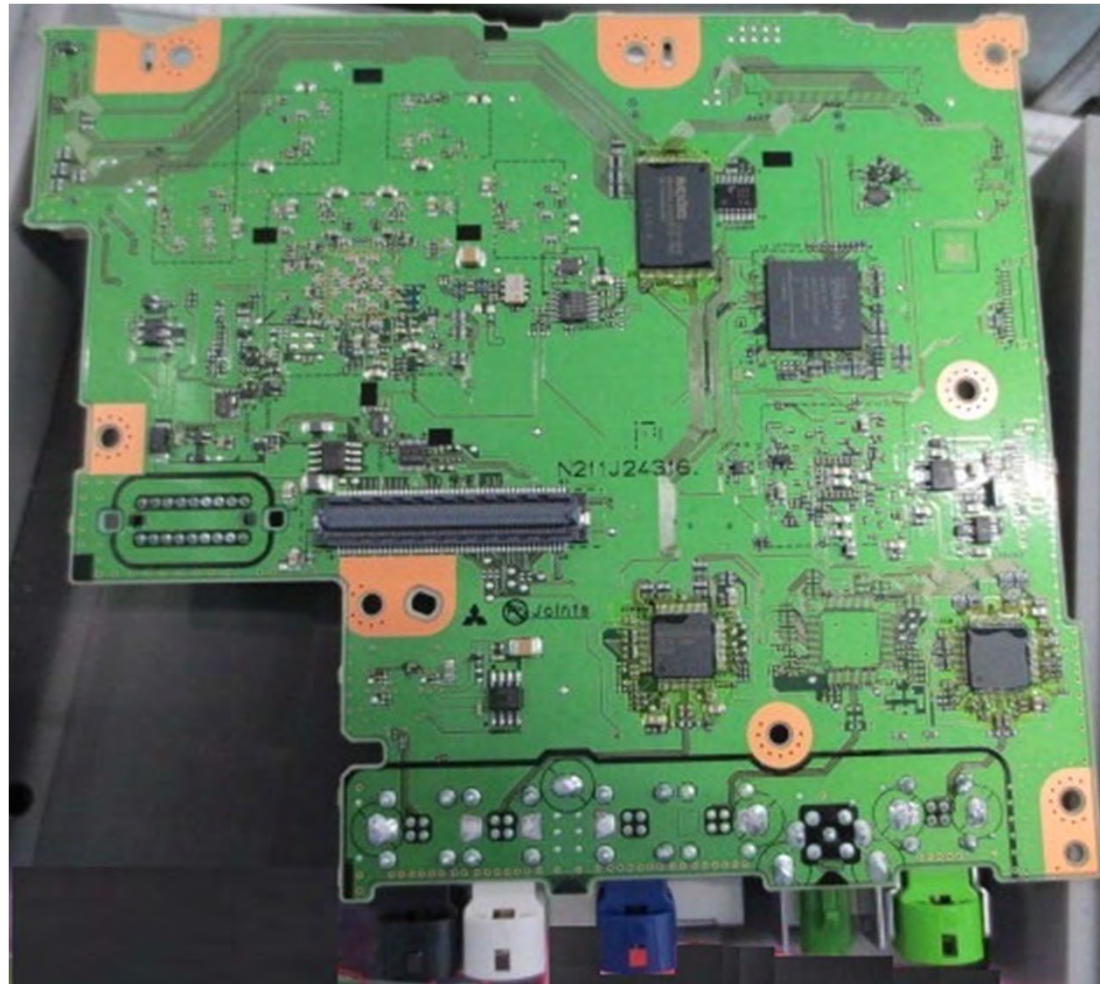
2. PCB-NAVI (PCB-NAVI-A) S-side
