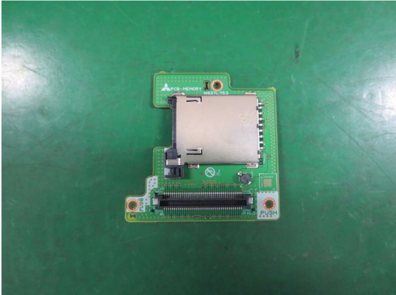
16. eSD-Module S-side
