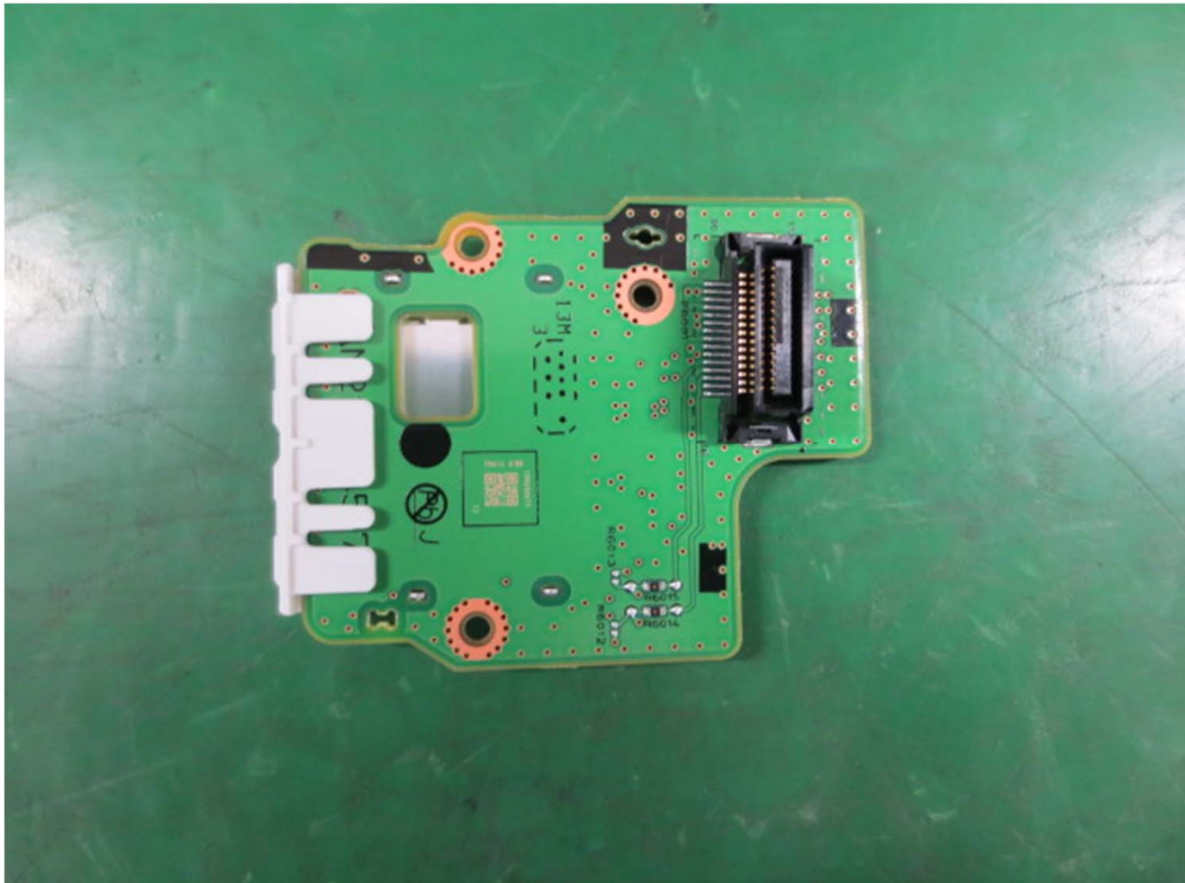
14. PCB-SD (PCB-NAVI-B) S-side
