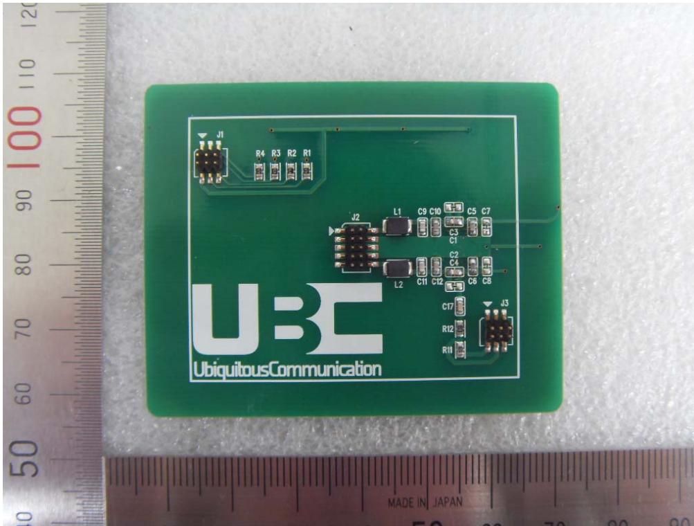
Antenna_RFID
