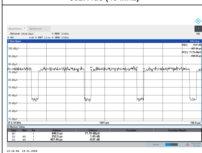
802.11ac (40 MHz)
