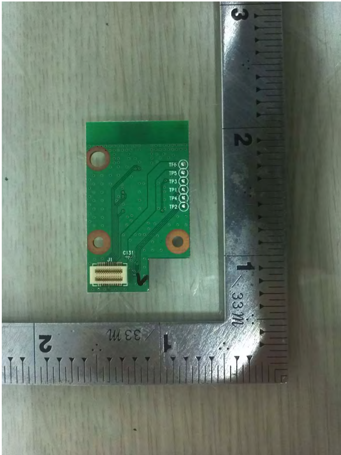
Bluetooth Module - Bottom
