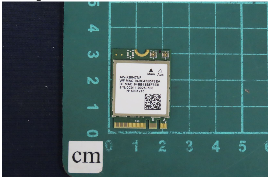
(4) EUT Photo _RTL8852BE
