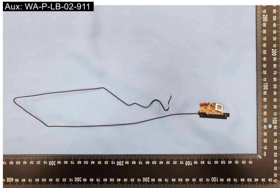
EUT Photo (14)
