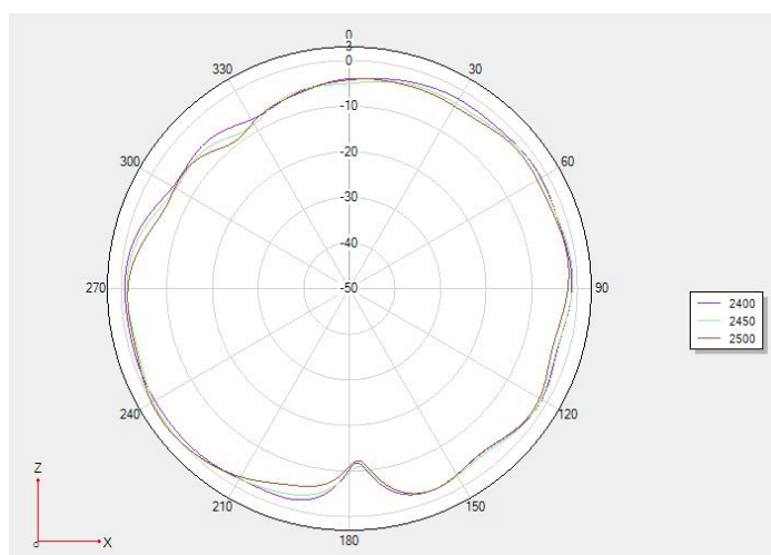
Phi 90 2D 图
