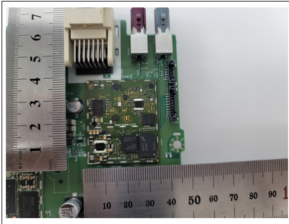
<CDMA/LTE Module>
