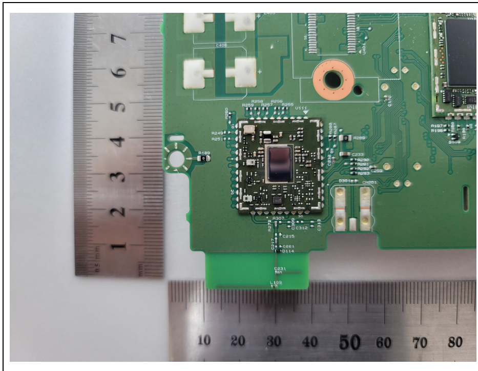
< BT Module >
