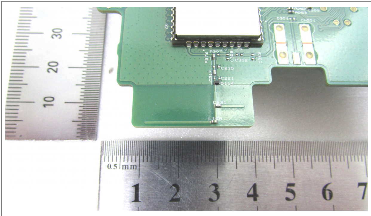
<WLAN Antenna>
