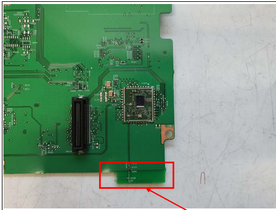
BT/WIFI Module
