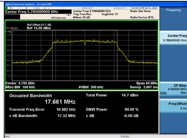
802.11ac(VHT20) (CH.157)
