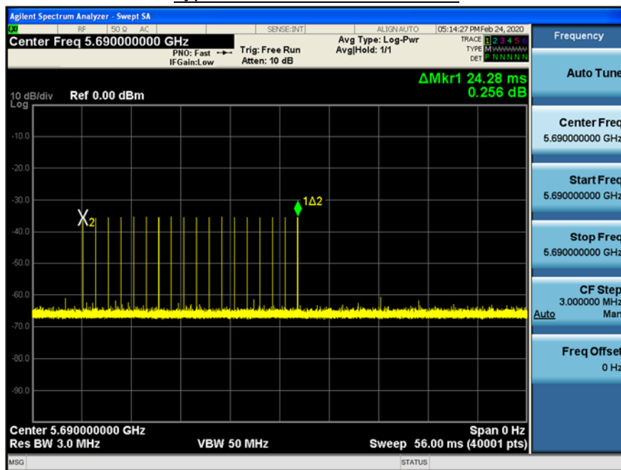
Type0 : PRI & Radar Pulse Number
