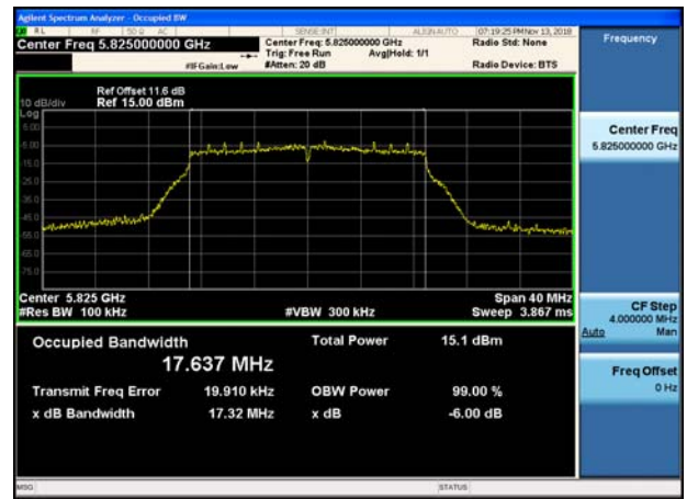
802.11ac(VHT20) (CH.165)
