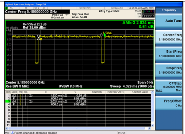
802.11ac(VHT20)
