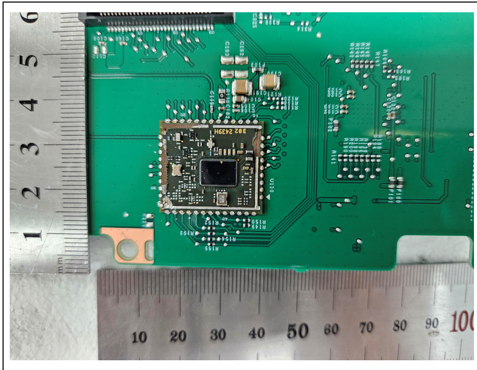
BT, WIFI Module
