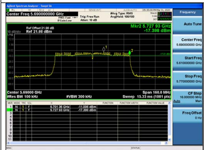
802.11ac_VHT80 CH.138
