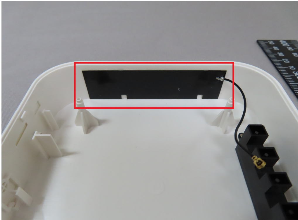
WWAN Antenna
