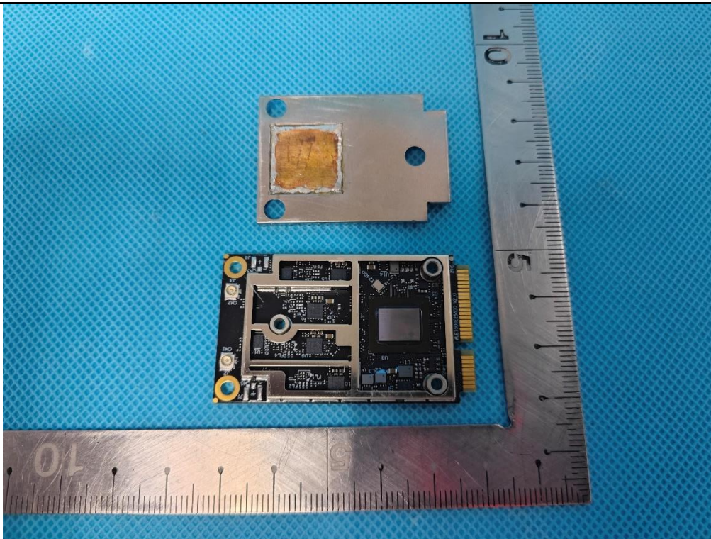
EUT Photo(6) - WLE7002E56
