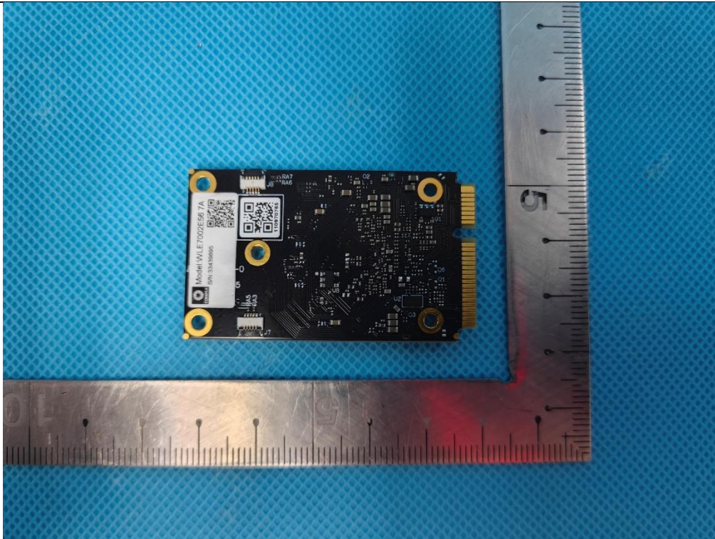
EUT Photo(8) - WLE7002E56
