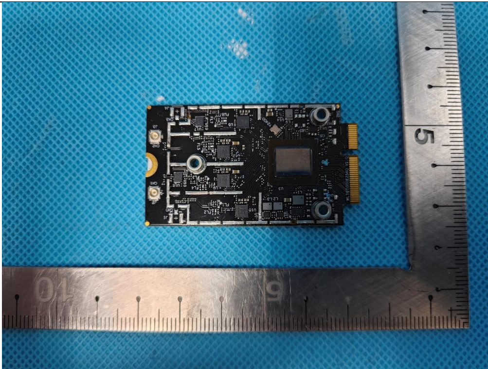
EUT Photo(12) - WLTE7002E56
