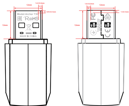
尺寸图
