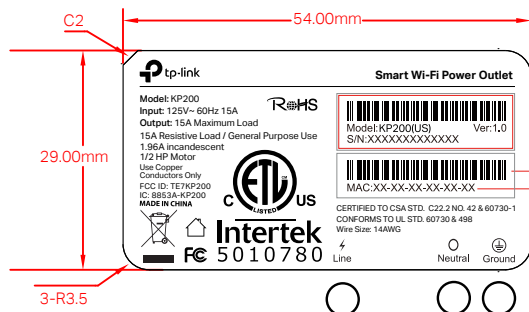
尺寸图 (54.00*29.00mm)
